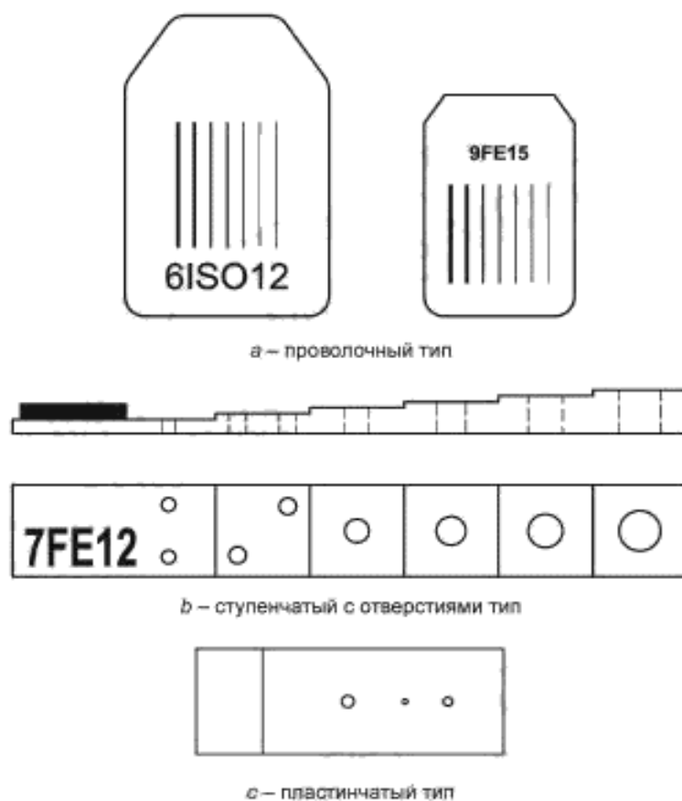
Рисунок 4 — Типы индикаторов качества изображения (IQI)
