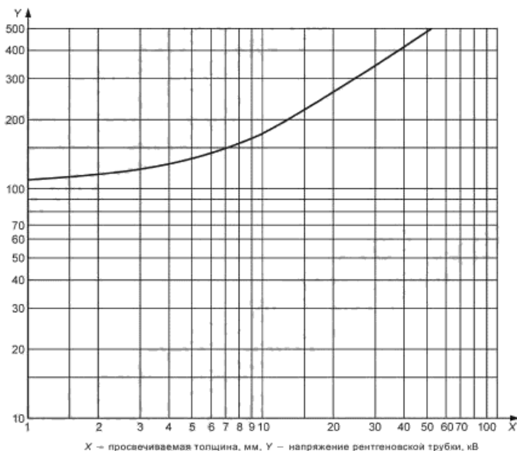
Рисунок 2 — Максимальное напряжение на рентгеновской трубке для аппаратов мощностью до 500 кВ как функция от просвечиваемой толщины
