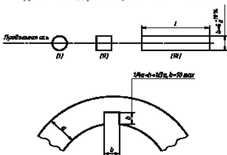
l — длина прямоугольной выемки (единственное ограничение l > 6 мм); b — ширина прямоугольной выемки и диаметр отверстий; h — глубина на прямоугольной выемки и отверстий; a — толщина стенки трубы
