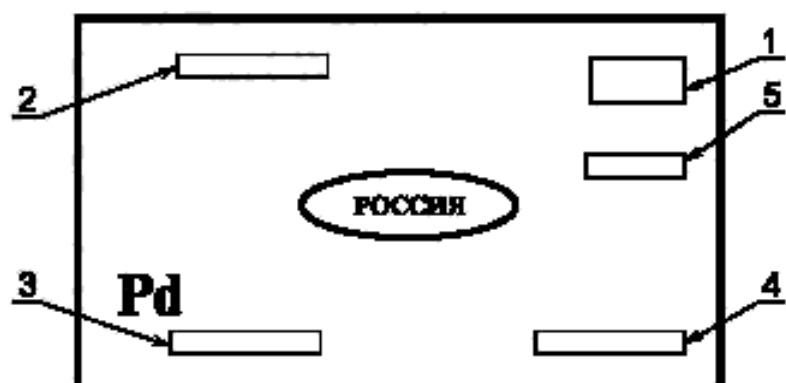
1 — товарный знак предприятия-изготовителя; 2 — номер (шифр) слитка; 3 — массовая доля палладия, %; 4 — масса слитка, г; 5 — год выпуска
