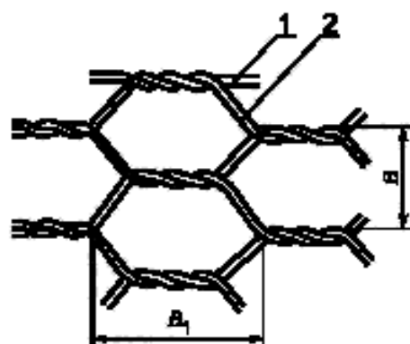
1 — проволока кромки; 2 — основная проволока; B — размер ячейки; B_1 — размер диагонали ячейки
