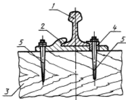
1 — рельс; 2 — подкладка полураздельного скрепления; 3 — шпала деревянная; 4 — шуруп; 5 — клемма специальная
