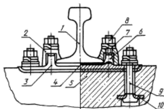
1 — рельс; 2 — клемма; 3 — подкладка раздельного скрепления; 4 — подрельсовая прокладка; 5 — прокладка под подкладку; 6 — клеммный болт; 7 — двухнитковая шайба; 8 — гайка; 9 — закладной болт; 10 — опорная шайба
