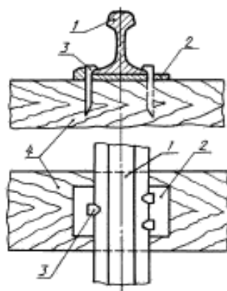
1 — рельс; 2 — подкладка нераздельного крепления; 3 — костыль путей; 4 — шпала деревянная
