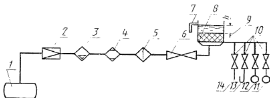
1—источник сжатого воздуха; 2—редукционный клапан; 3—влажномаслоотделитель; 4—осушитель; 5—фильтр; 6—кран точной регулировки; 7—сливная трубка для установки уровня жидкости над образцом; 8—испытываемый образец; 9—держатель для крепления образцов; 10—кран; 11—манометр Мо 0,4 МПа по ГОСТ 6521—72; 12—манометр Мо 0,16 МПа по ГОСТ 6521—72; 13—U-образный манометр, заполненный водой; 14—микроманометр ММН-2400(5)—0,6 ГОСТ 11161—84.
