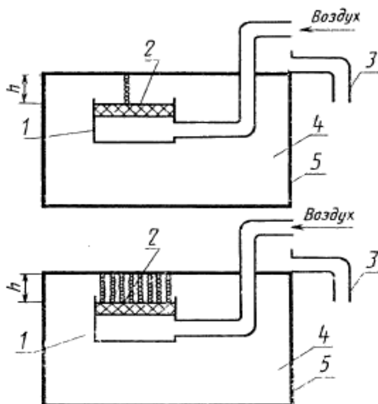
1—держатель образца; 2—испытуемый образец; 3—трубки для слива жидкости; 4—жидкость; 5—сосуд для жидкости; h —высота столба жидкости над испытуемым образцом.
