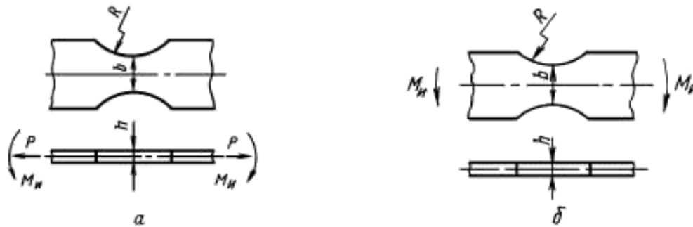
Рабочая часть образца типа III
