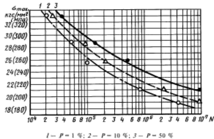
Кривые усталости образцов из сплава марки В95
