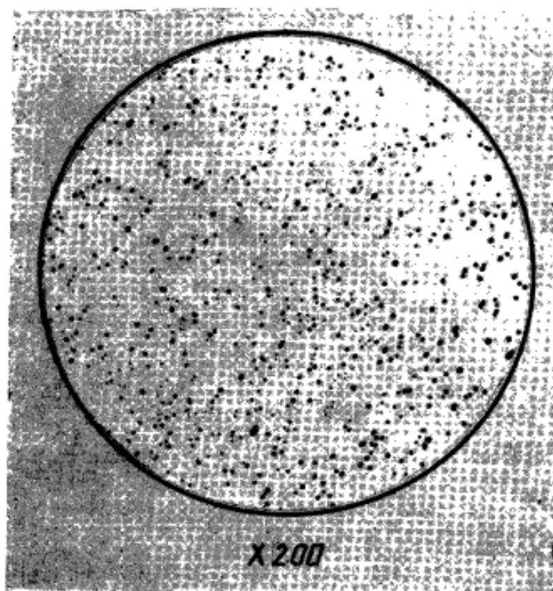
Черт. 4. Материал — деформированная медь, массовая доля кислорода — 0,09%, освещение — рассеянный свет
