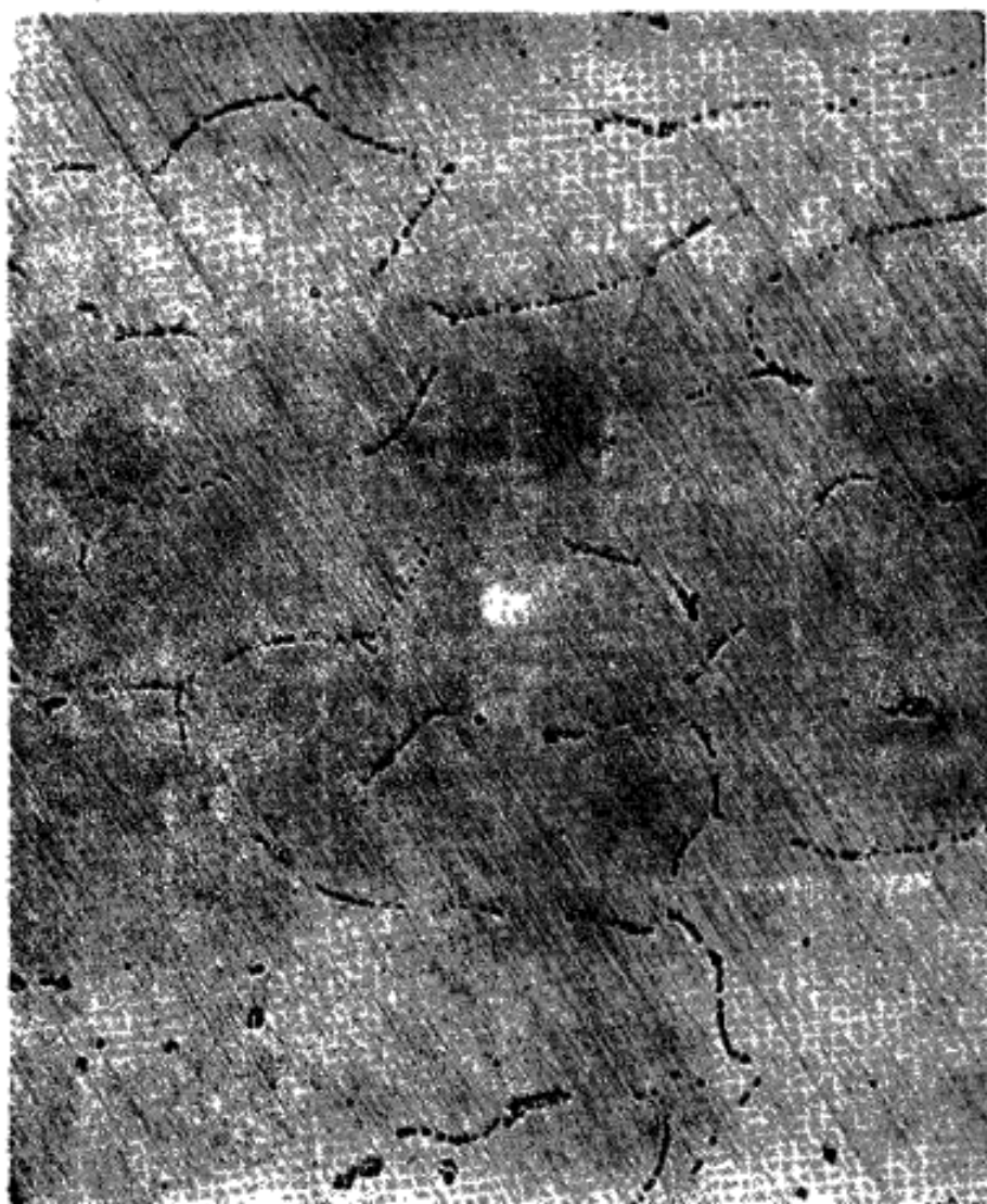
Черт. 8. Материал — литая медь, массовая доля кислорода — 0,022%, освещение — рассеянный свет
