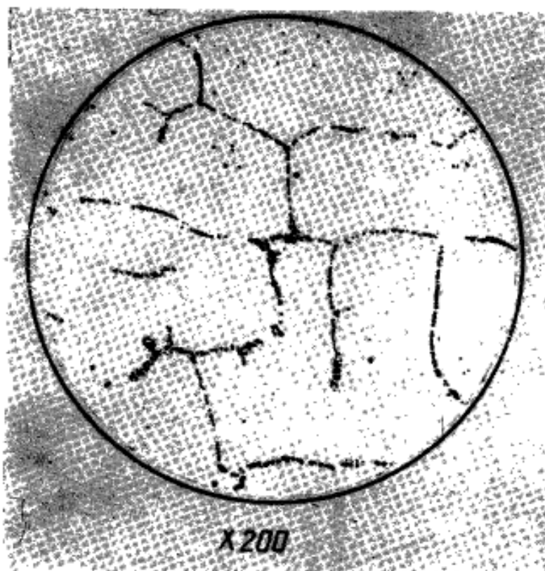
Черт. 9. Материал - литья медь, массовая доля кислорода — 0,035%, освещение — рассеянный свет
