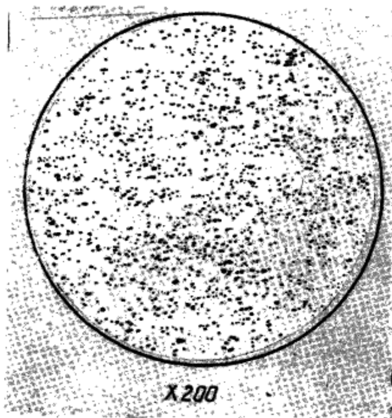
Черт. 5. Материал — деформированная медь, массовая доля кислорода — 0,12%, освещение — рассеянный свет
