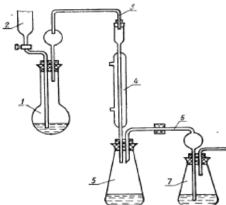
1—перегонная колба вместимостью 500 см 3 ; 2—капельная воронка; 3—насадка с брызгоуловителем; 4—водяной холодильник; 5—приемник (коническая колба вместимостью 250 см 3 ); 6—стеклянная трубка с грушевидным расширением; 7—контрольный приемник (коническая колба вместимостью 250 см 3 )
