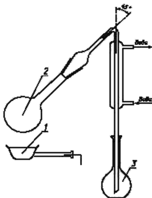
1 — нагреватель мощностью 300 Вт; 2 — круглодонная колба вместимостью 500 см 3 ; 3 — мерная колба с при- шлифованным горлом вместимостью 100 см 3
