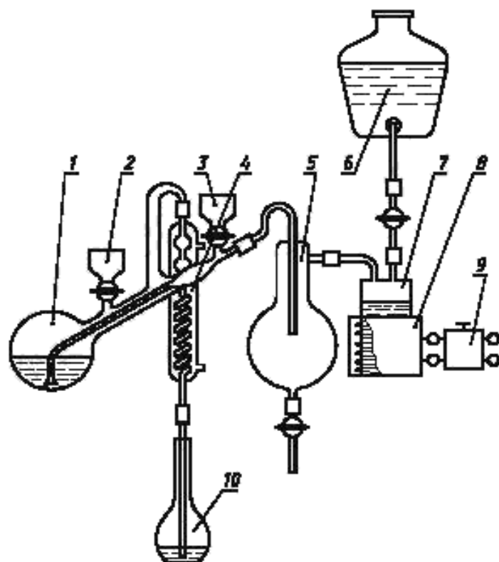
Рисунок 1 — Схема установки для дистилляции аммиака с паром
