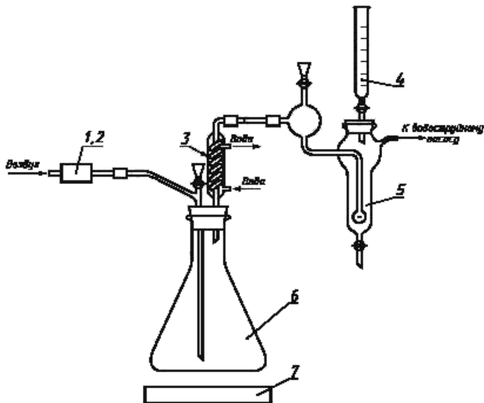
Рисунок 3 — Схема установки для дистилляции аммиака с воздушной аспирацией
