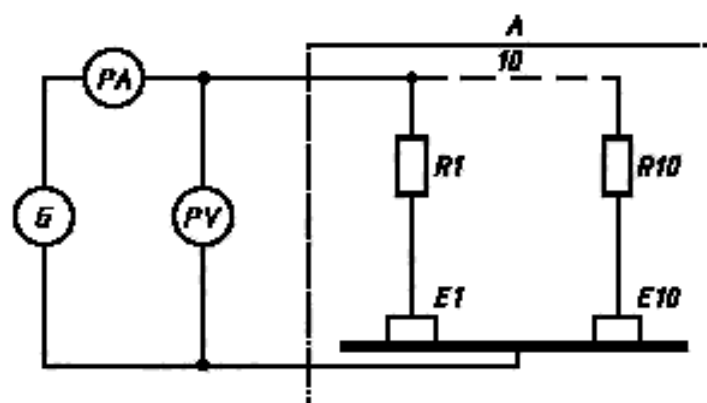
Рисунок 1 — Схема для измерения сопротивления изоляционного покрытия
